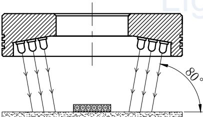
照明示意图
