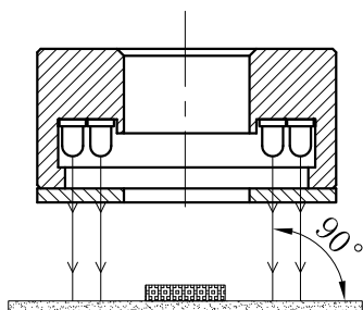
照明示意图
