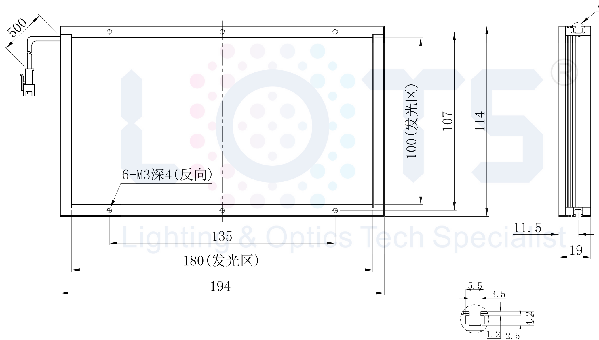
视图A，比例2:1
